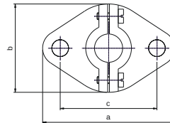
Flange DIN 43734 Cast iron
